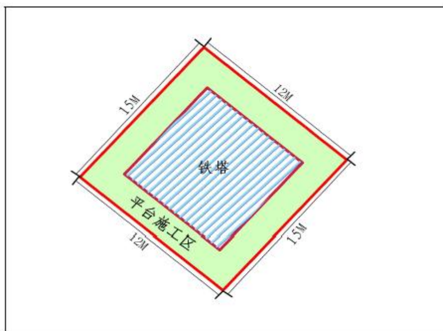
图 2-7 铁塔吊装平台平面布局图
