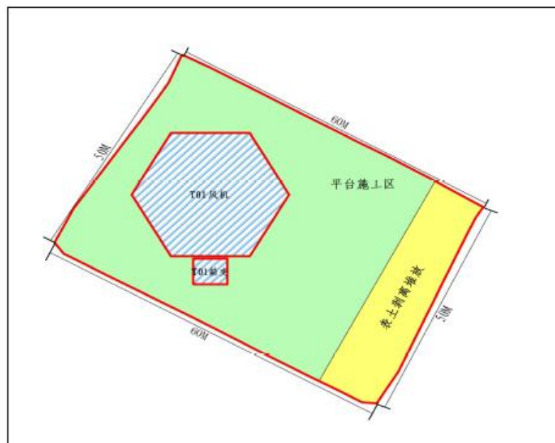
图 2-6 风机吊装平台平面布局图
