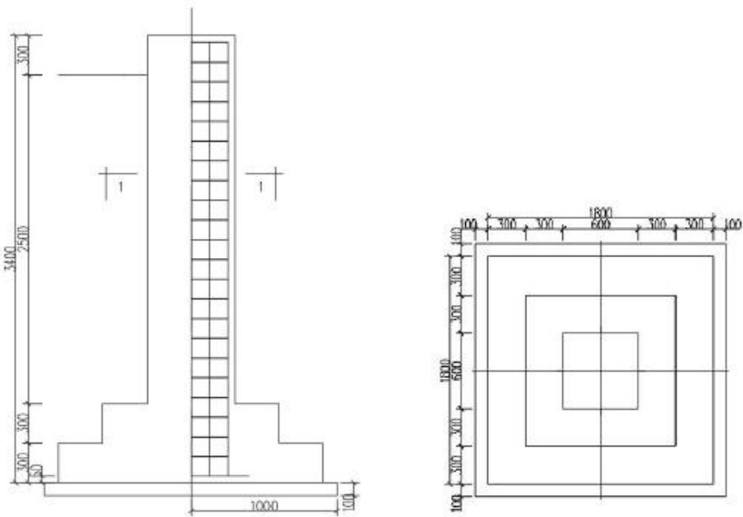
图 2-3 直线塔基础型式图
