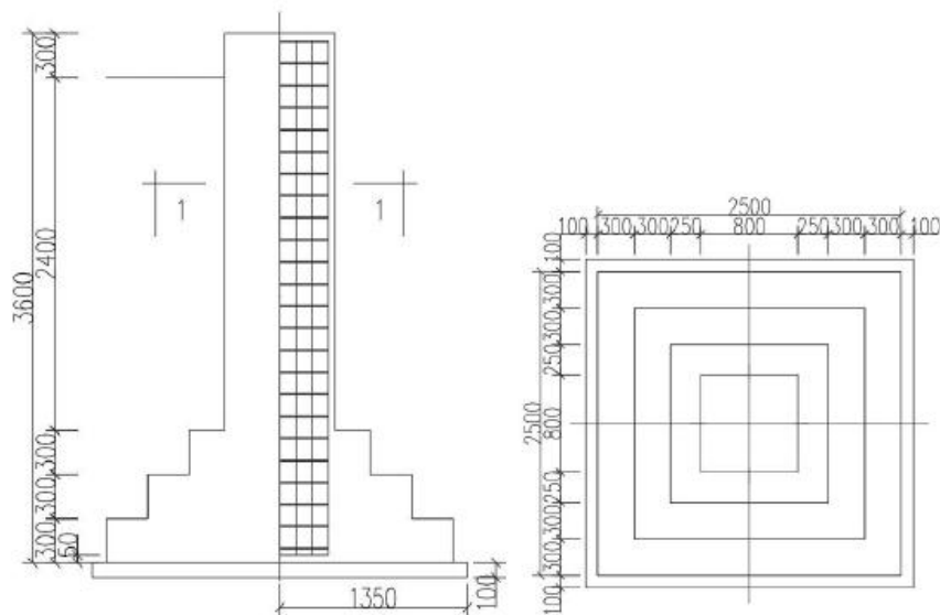
图 2-4 耐张塔基础型式图
