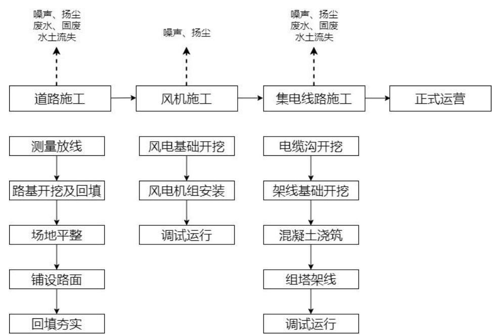
图 2-4 施工工艺流程图
